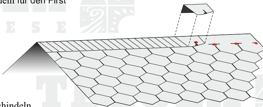
Abb. 7 - Schneiden der Schindeln für den First
